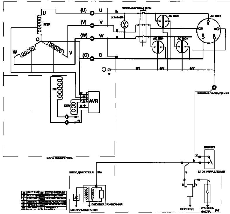
ЭЛЕКТРИЧЕСКАЯ СХЕМА
